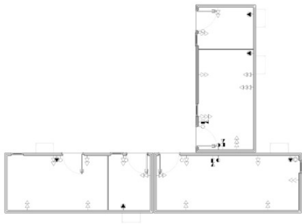
3 Térreo - Executivo PONTOS ELÉTRICOS 1 : 75
