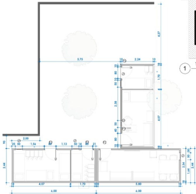
2 Térreo - Executivo 1 : 75
